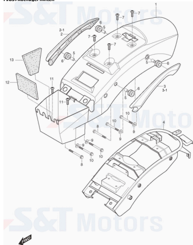
FIG37Kotflügel hinten
