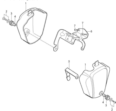
FIG17Verkleidungsdeckel
