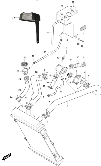
FIG16 Kühlerschläuche & Ausgleichsbehälter
