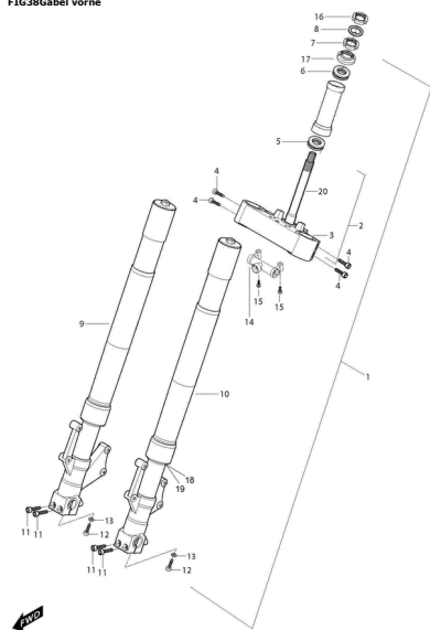
FIG38Gabel vorne
