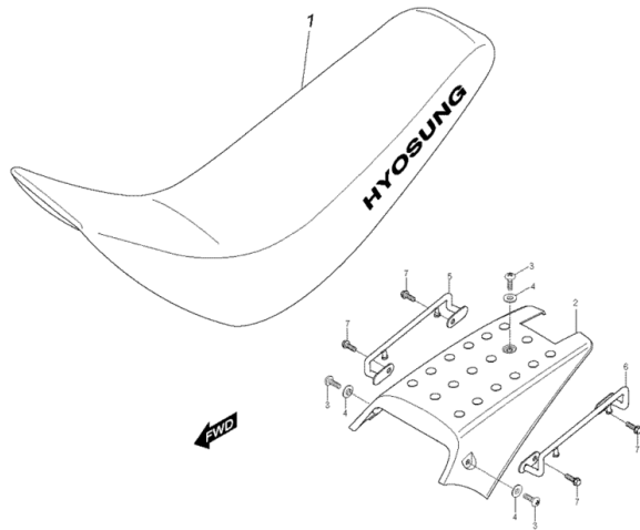
FIG33Sitz / Bordwerkzeug
