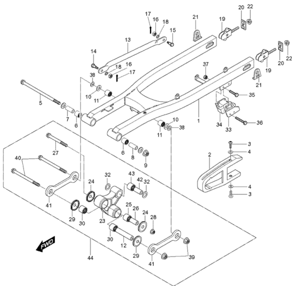
FIG41 Schwinge hinten
