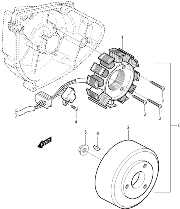
FIG19Lichtmaschine
