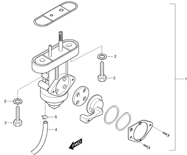
FIG32Benzinhahn
