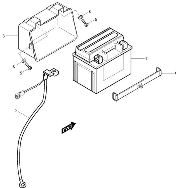
FIG20Batterie
