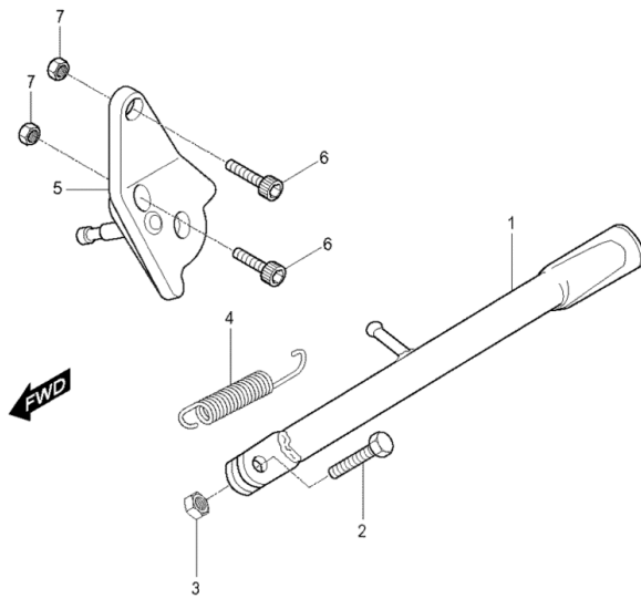
FIG28Seitenständer
