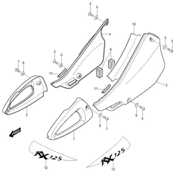
FIG34Verkleidungen hinten
