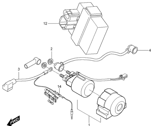
FIG21 Elektrik
