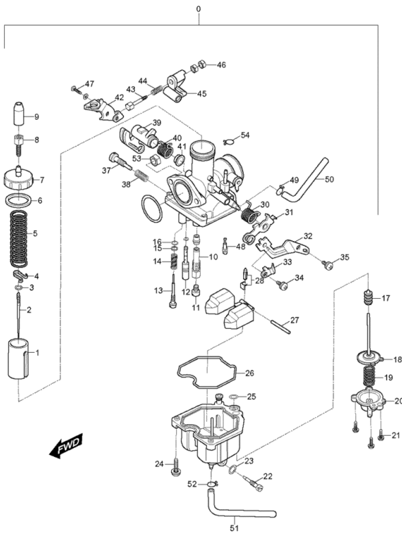
FIG10Vergaser
