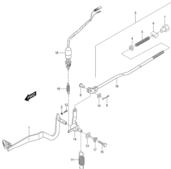
FIG29Bremsgestänge hinten
