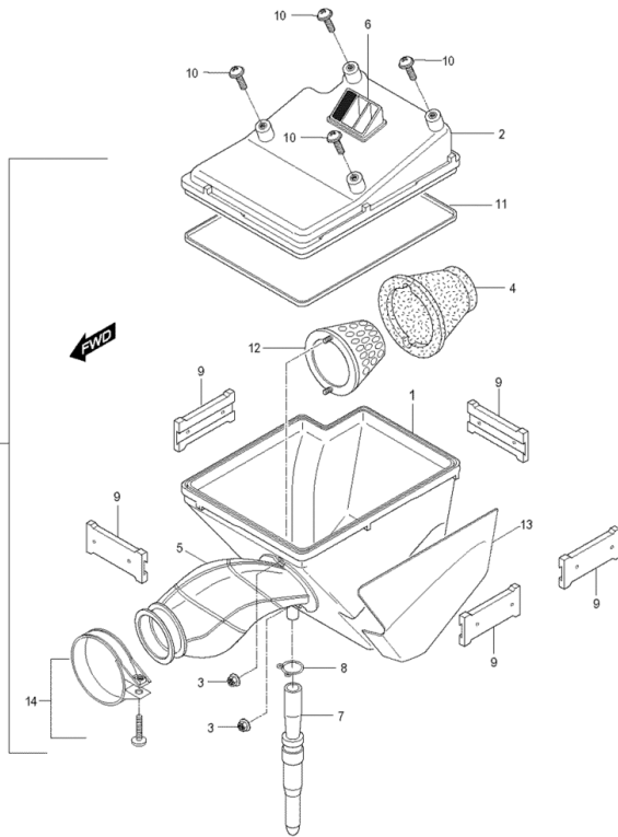
FIG11 Luftfilter
