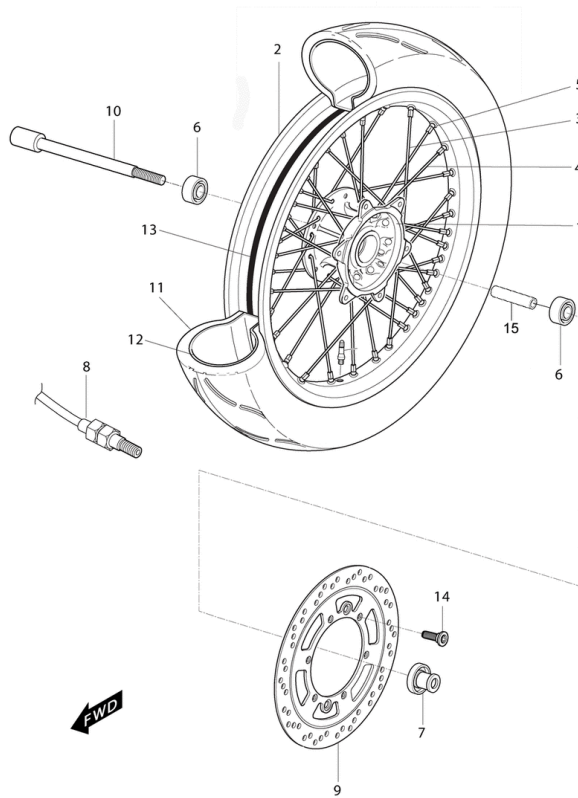
FIG35Vorderrad
