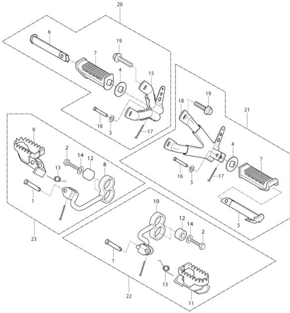
FIG29Fussrasten vorn & hinten
