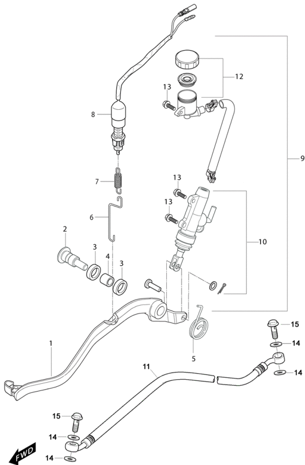
FIG28Fussbremspedal
