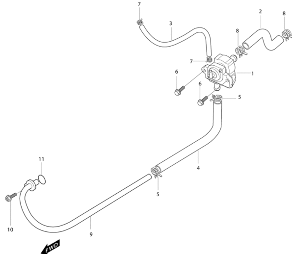
FIG13Sekundärluftventil
