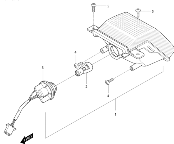
FIG24Rücklicht
