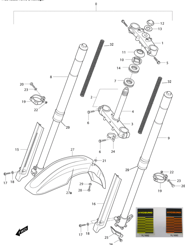
FIG34Gabel vorne & Kotflügel
