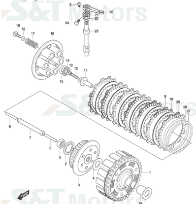
FIG18Kupplung
