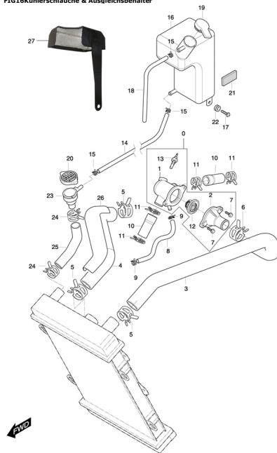
FIG16 Kühlerschläuche & Ausgleichsbehälter
