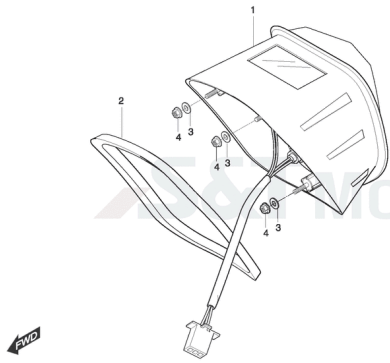
FIG29Rücklicht
