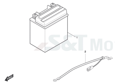
FIG23Batterie
