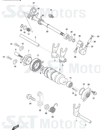
FIG20Schaltung
