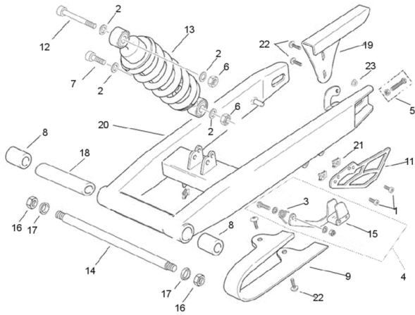
FIG32Schwinge, Federbein hinten
