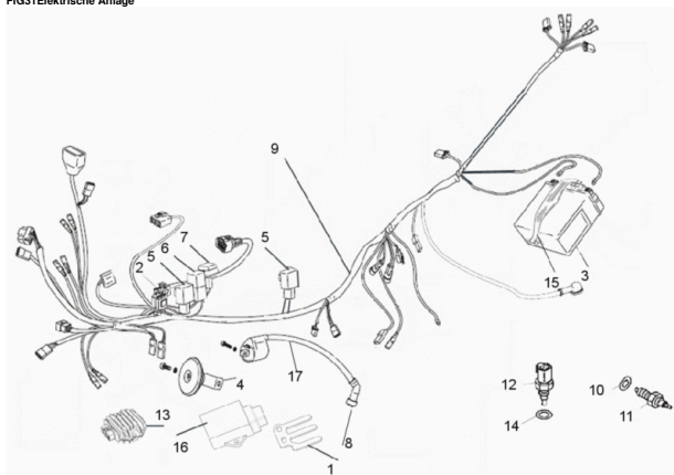
FIG31 Elektrische Anlage
