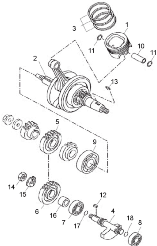
FIG05Kolben, Pleuellwelle, Ausgleichswelle
