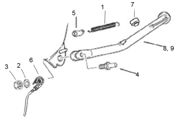
FIG33Seitenständer, Seitenständerschalter
