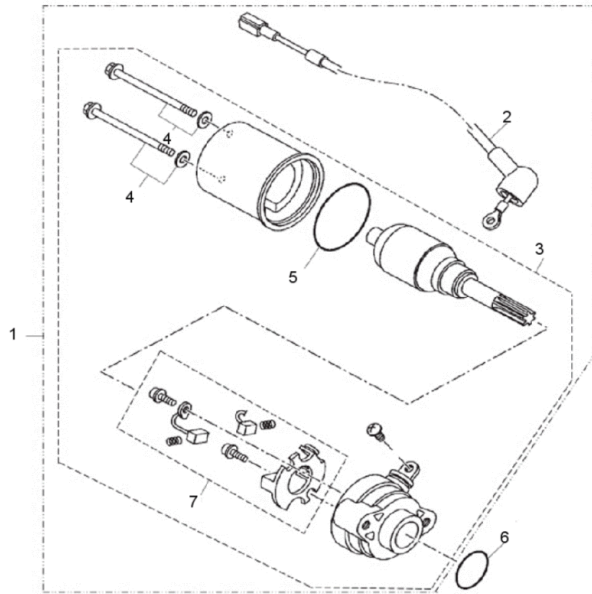
FIG14 Anlasser
