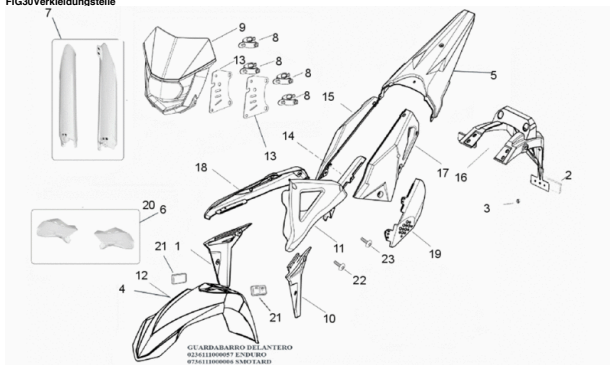
FIG30 Verkleidungsteile
