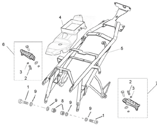
FIG35Rahmenheck, Fußrasten
