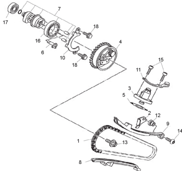
FIG07Nockenwelle, Steuerkette
