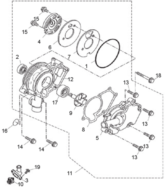
FIG12 Wasserpumpe
