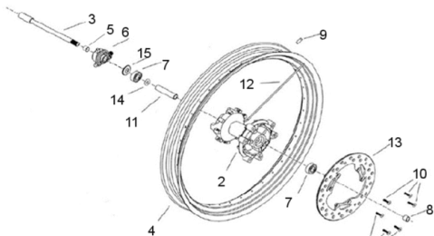
FIG23a Enduro Vorderrad, Bremsscheibe
