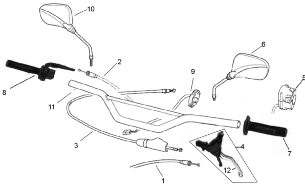
FIG21Lenker, Spiegel, Bowdenzüge, Kombischalter
