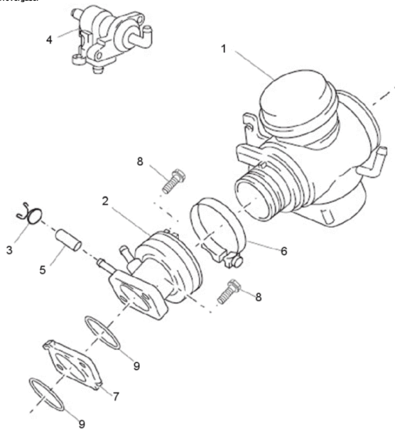
FIG16Vergaser
