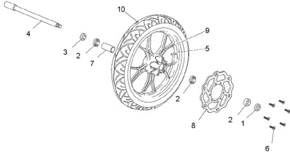
FIG23 Supermoto Vorderrad, Bremsscheibe
