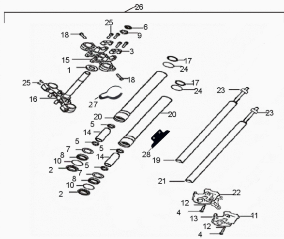
FIG22Gabel vorne
