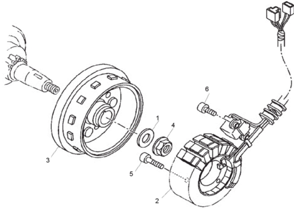
FIG13 Lichtmaschine
