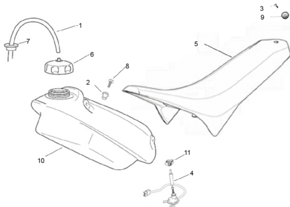
FIG29 Tank, Benzinhahn, Sitzbank
