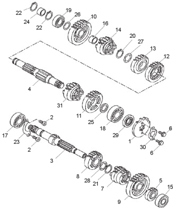
FIG10Getriebe
