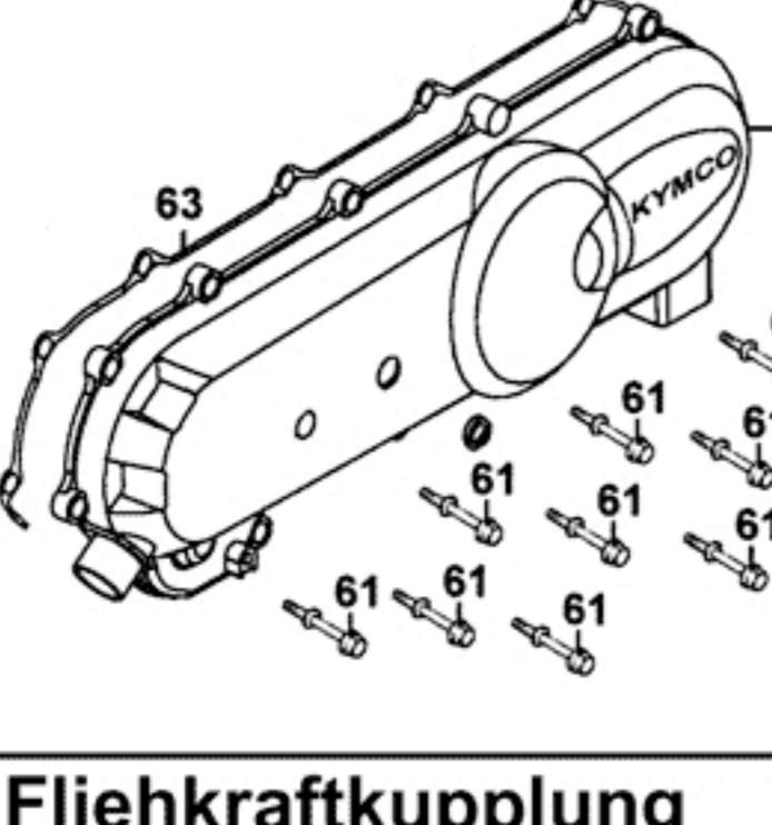
E07 Fliehkraftkupplung Hi. Antrieb
