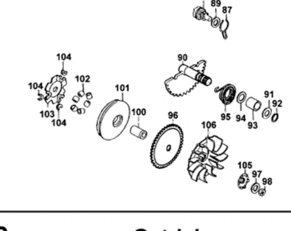
E08 Getriebe
